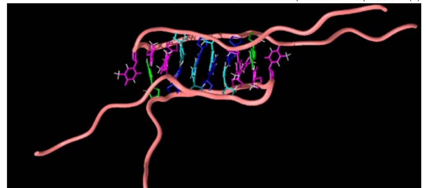
Estructura no-canónica ("i-motif") de ADN formada por secuencias del centrómero humano. Estructura tridimensional obtenida en disolución a partir de datos de RMN adquiridos en el LMR (46).
