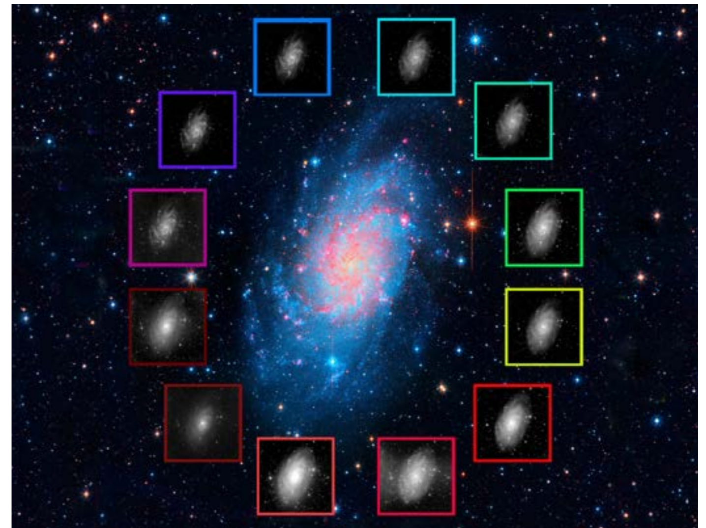
Imagen de la galaxia M33 en color y en los 12 filtros de J-PLUS. Crédito: CEFGA.
