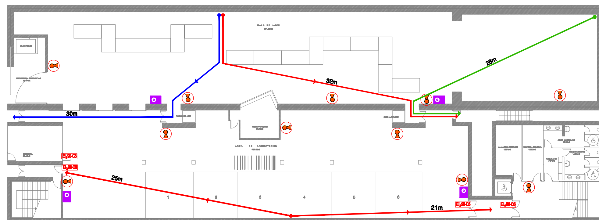
PLANTA SEMISÓTANO
