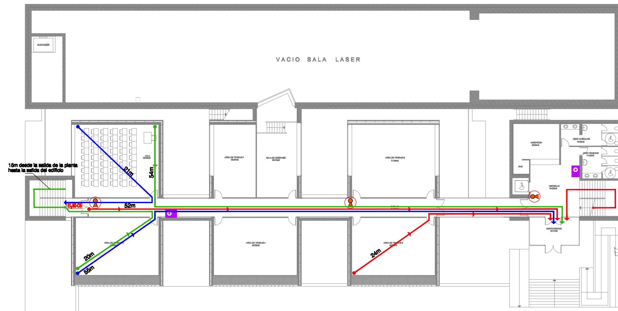
PLANTA BAJA
